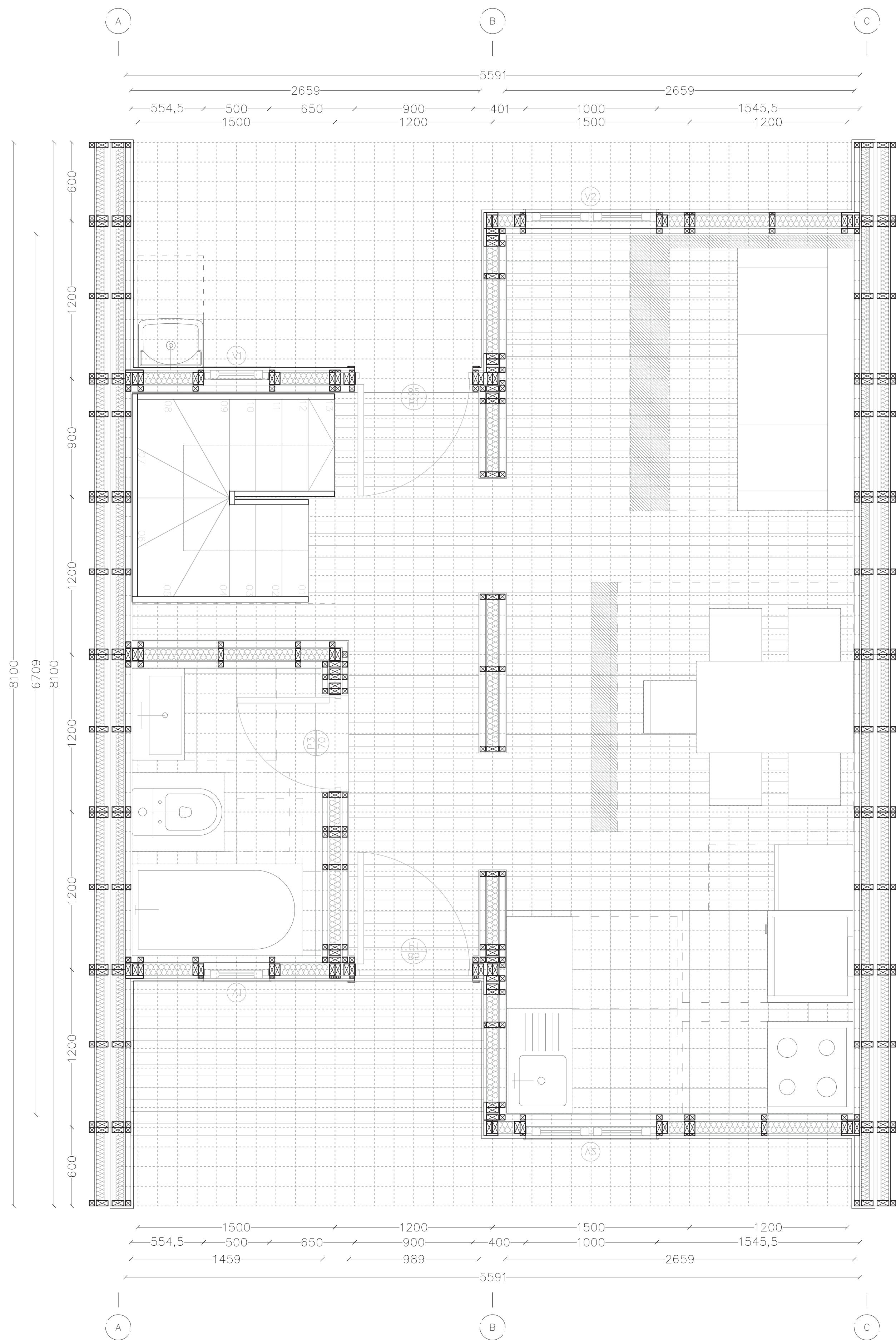
Planta primer nivel | "Vivienda d.s 49 tipología continua" Escala 1:20
