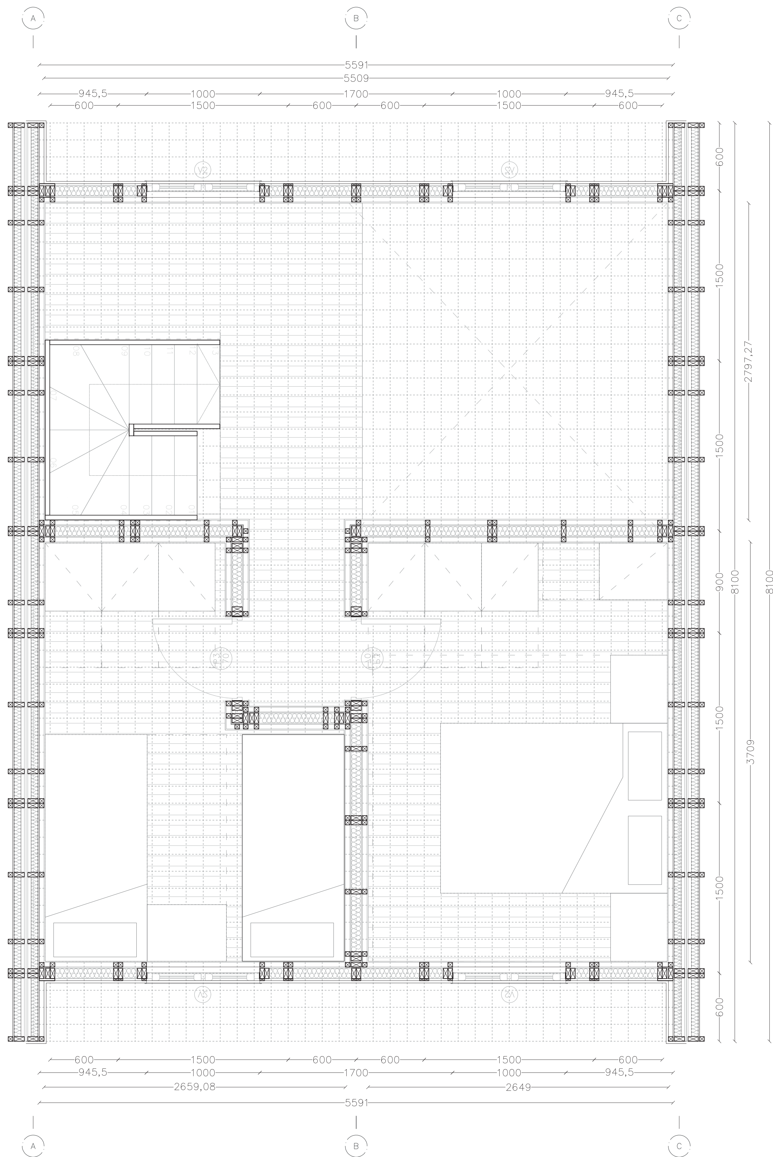
Planta segundo nivel | "Vivienda d.s 49 tipología continua" Escala 1:20
