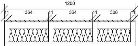
Elevación
