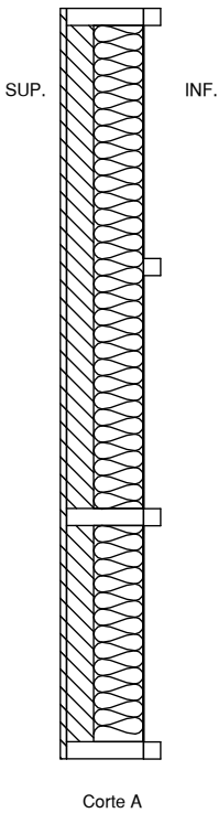
Corte A
