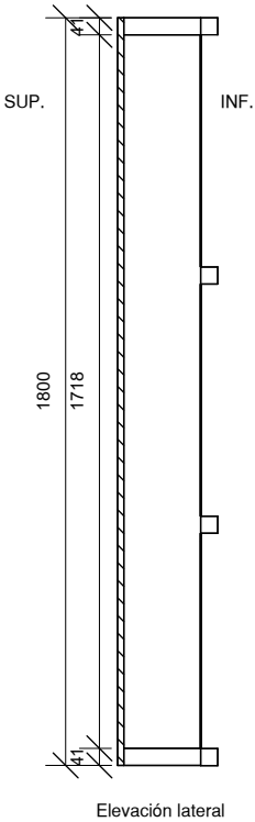
Elevación lateral
