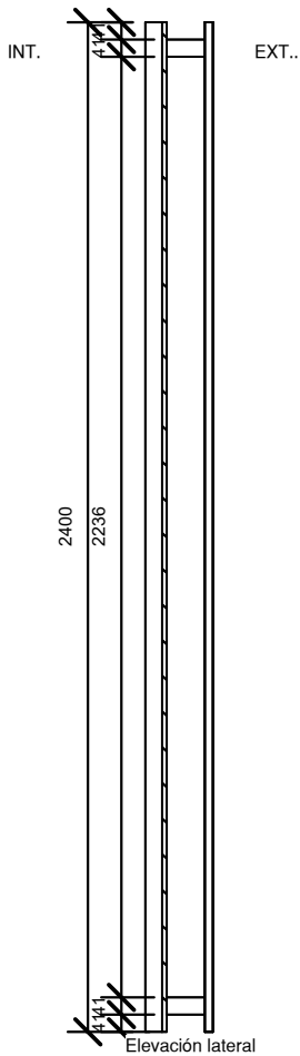
Elevación lateral
