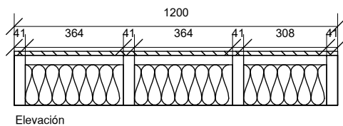
Elevación
