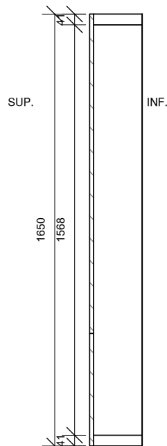
Elevación lateral
