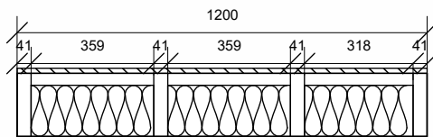
Elevación
