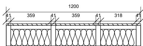
Elevación
