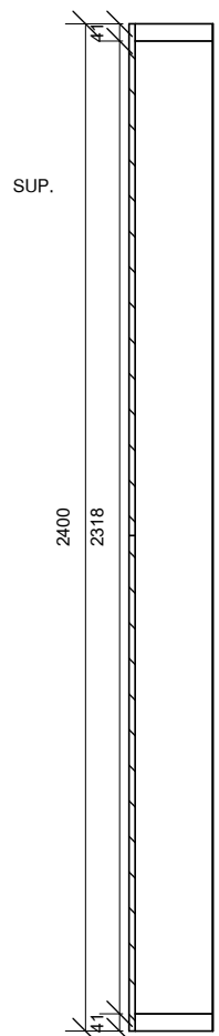
Elevación lateral
