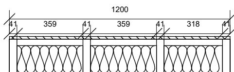
Elevación
