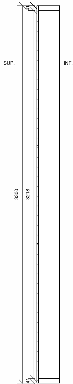
Elevación lateral
