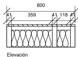
Elevación
