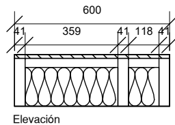
Elevación
