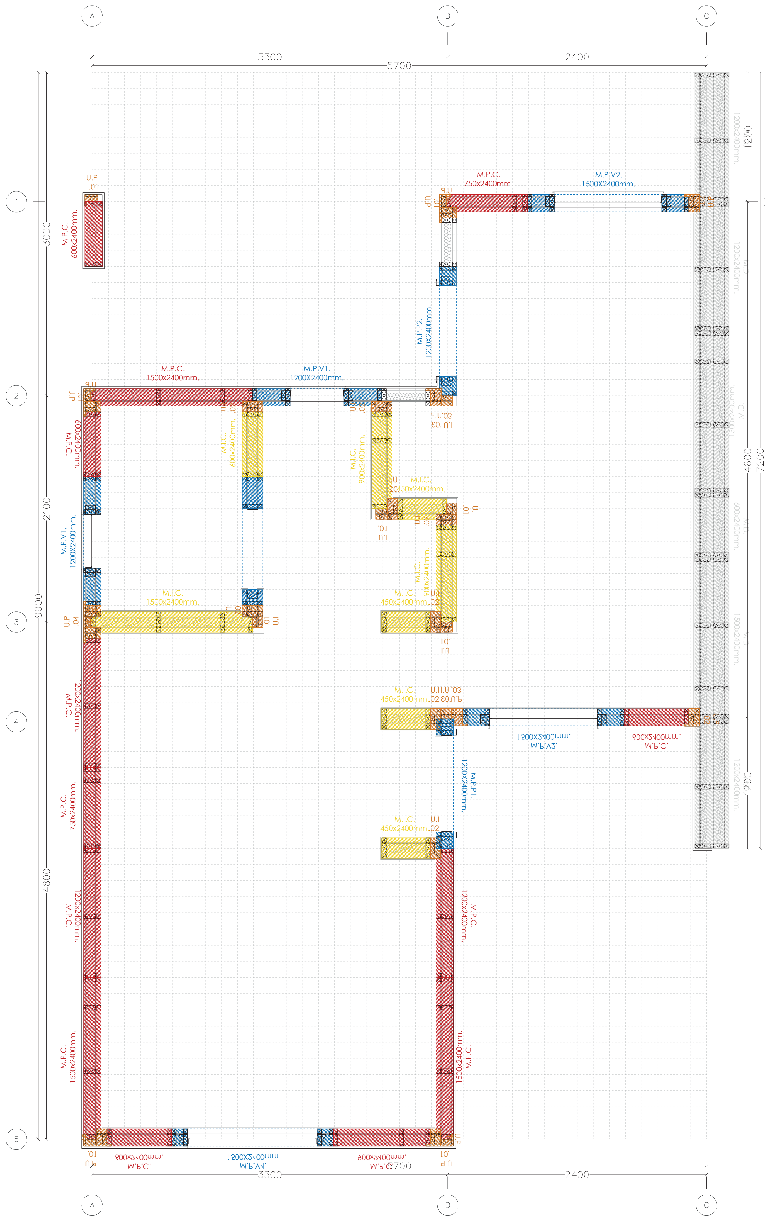
Planta primer nivel componenetes de muros | "Vivienda d.s 49 tipología pareada" Escala 1:20
