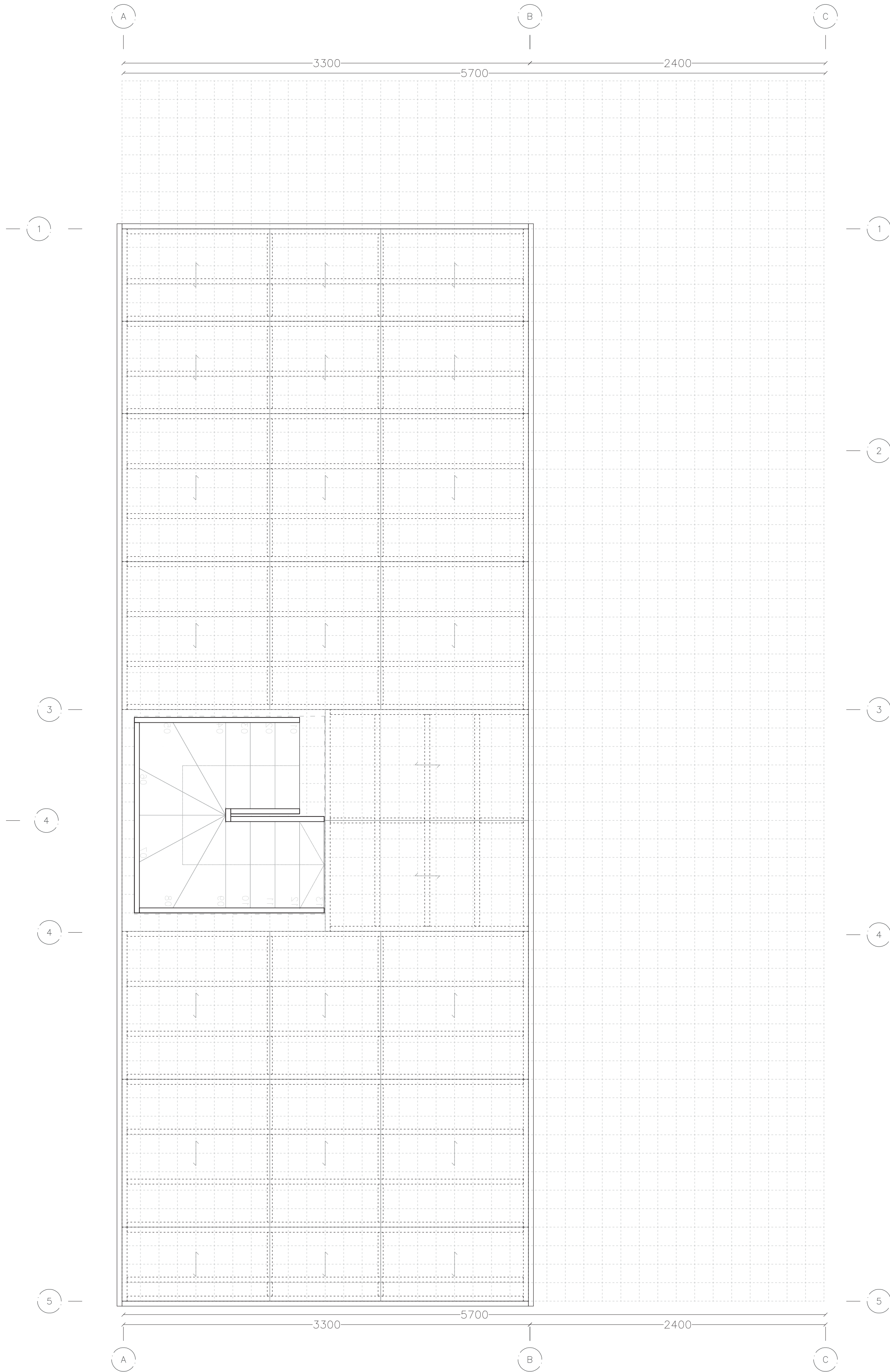
Planta Entrepiso | "Vivienda d.s 49 tipología pareada" Escala 1:20
