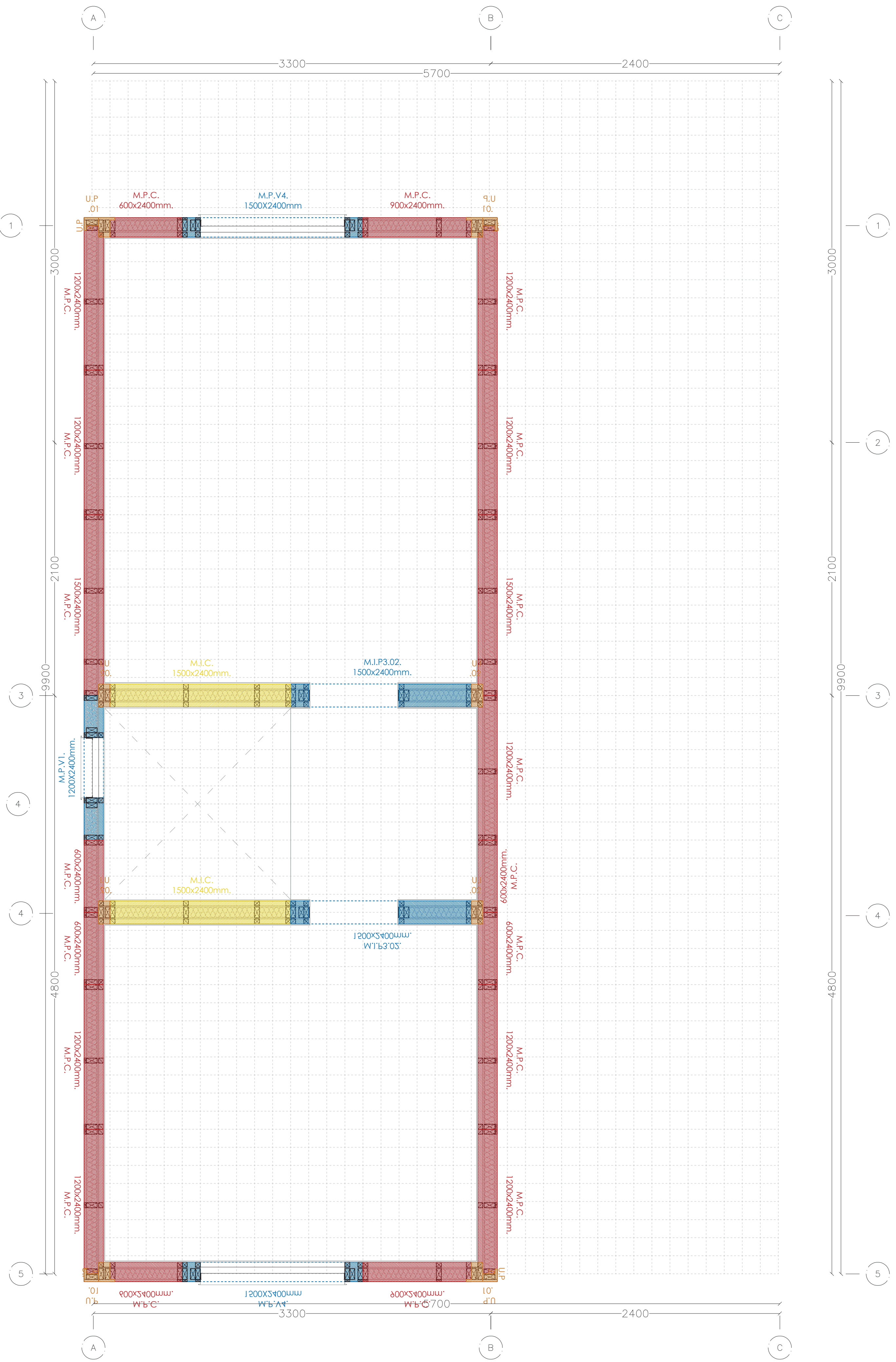
Planta segundo nivel componenetes de muros | "Vivienda d.s 49 tipología pareada" Escala 1:20
